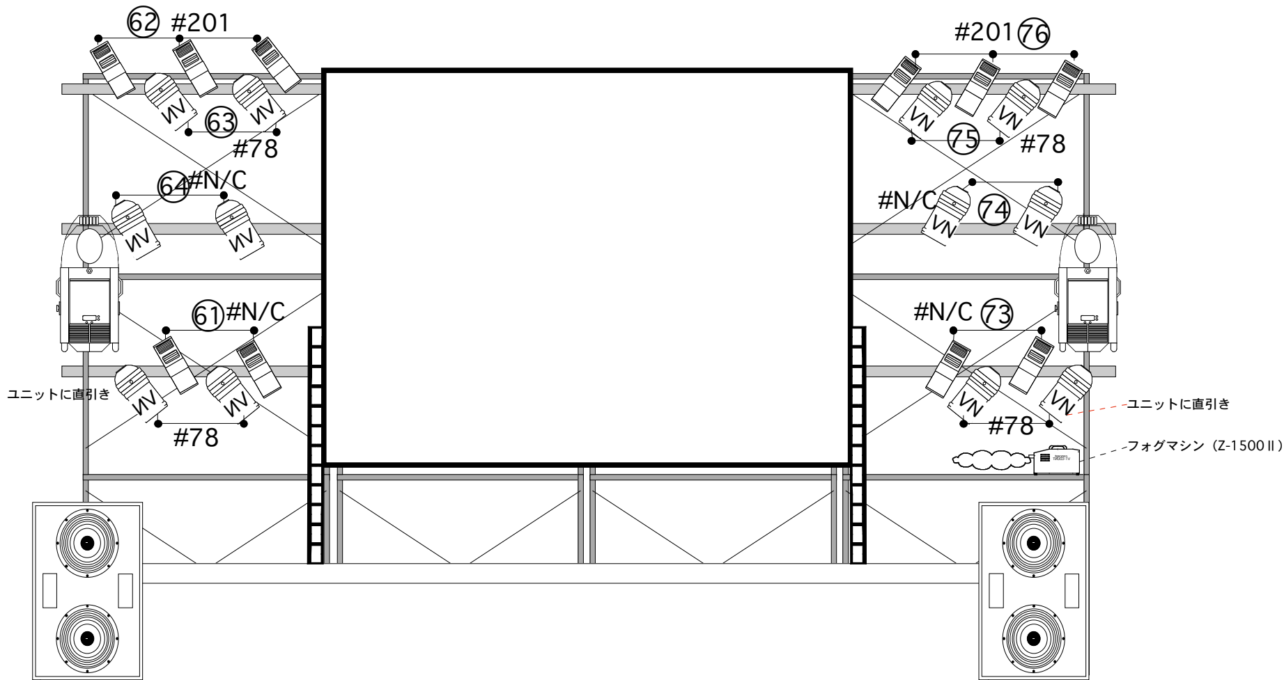
ステージバックにA1イントレ3段×4スパン設置
